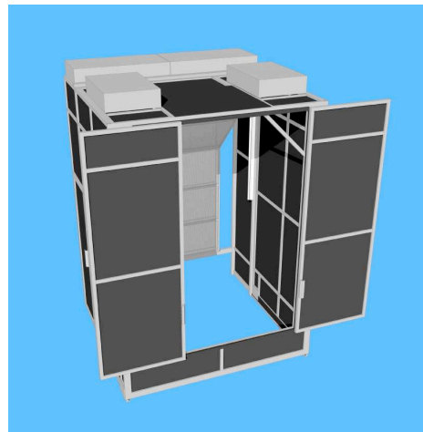
Individuelle Einhausung customized Minienvironment
